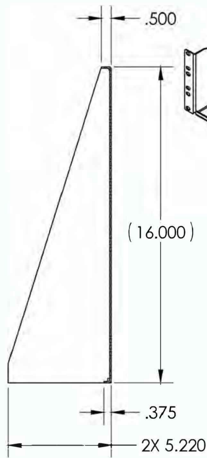
SECTION A-A
