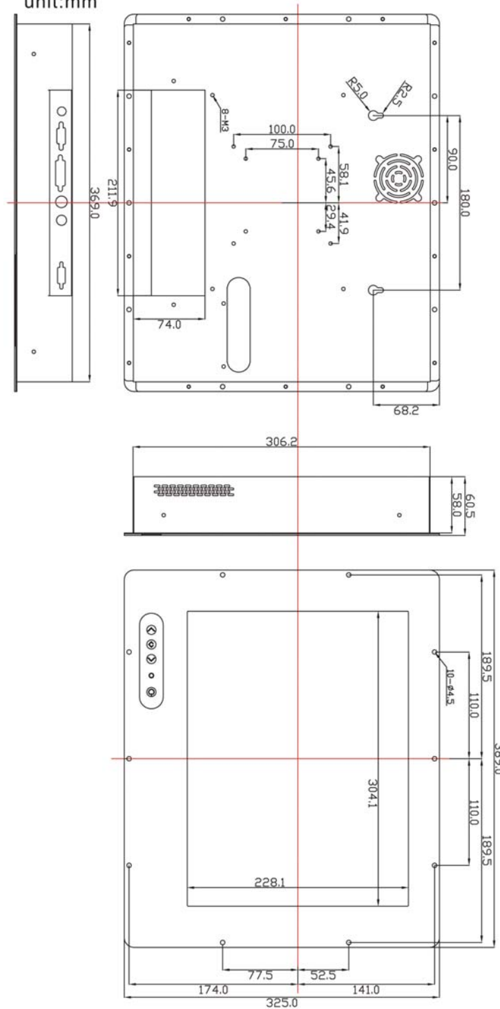
Outline Dimensions unit:mm
